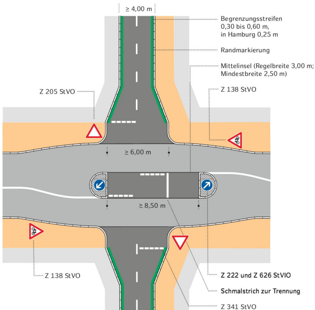
Abb. 5.9 Schaubild Musterlösung S4 innerorts (Quelle: PGV-Alrutz)
