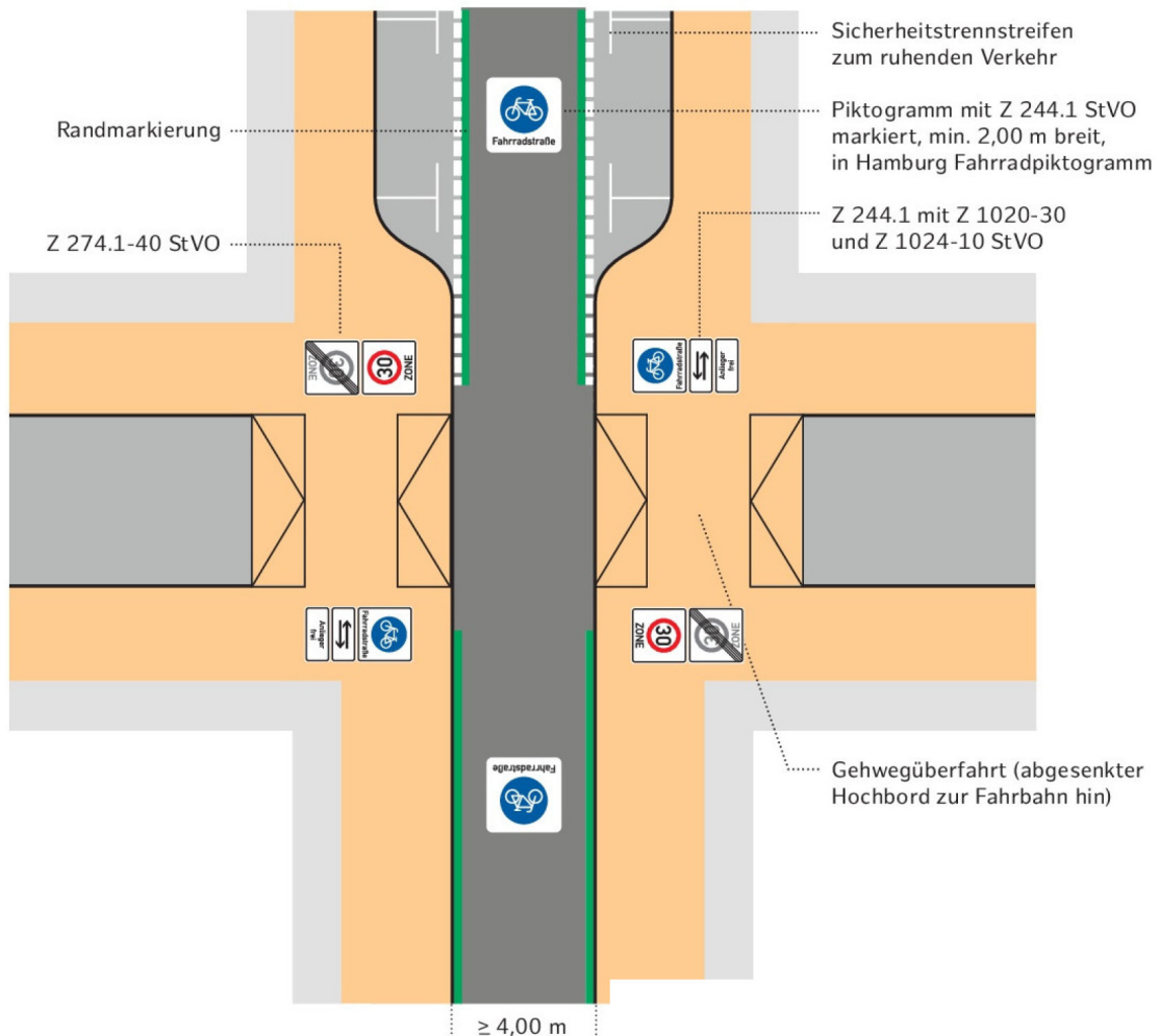
Abb. 5.10 Schaubild Musterlösung N1 (Quelle: PGV-Alrutz)
